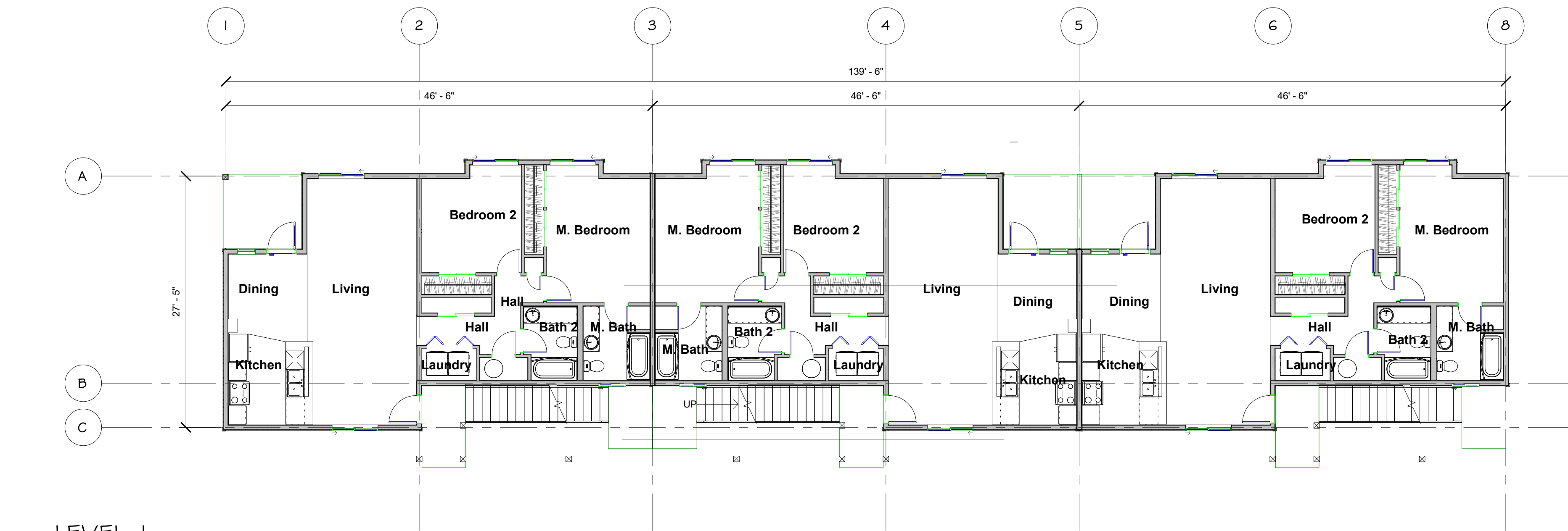
1 LEVEL 1 SCALE: 1/8" = 1'-0"
